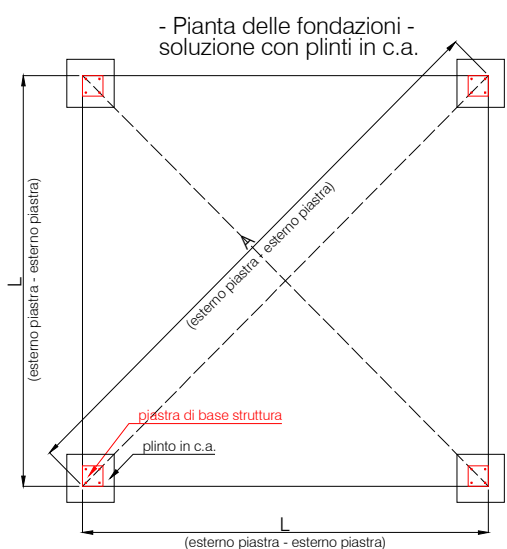
Dimensioni e peso dei plinti/zavorre necessarie per ogni piantone
